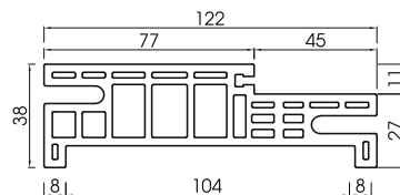
Đố cửa 120 - PWF120 Door frame 120 - PWF120
