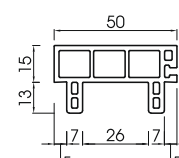
U đố cửa 100H - PW 050 Door frame cap 100H - PW 050
