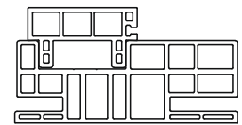
Bộ đố cửa 100H Door frame set 100H
