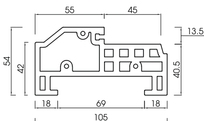
Đố cửa 105 - PAK105 Door frame 105 - PAK105
