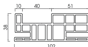
Đố cửa 100H - PWF100H Door frame 100H - PWF100H
