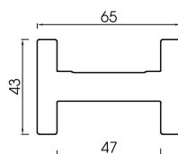
Thanh ray PABT 6543 Sliding door rail PABT 6543
